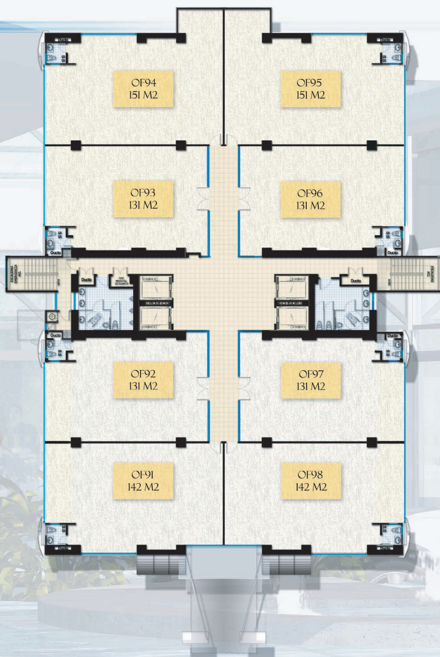
PLANTA DE DISTRIBUCION ARQUITECTONICA OFICINAS PISO 9
