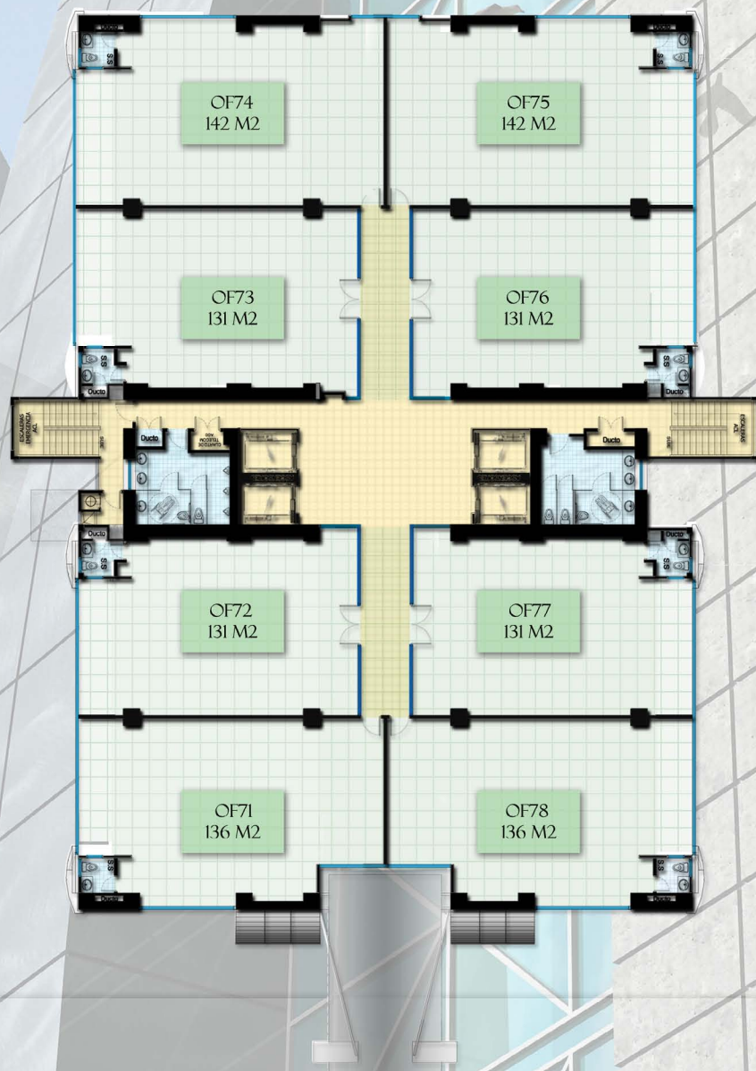
PLANTA DE DISTRIBUCION ARQUITECTONICA OFICINAS PISO 7
