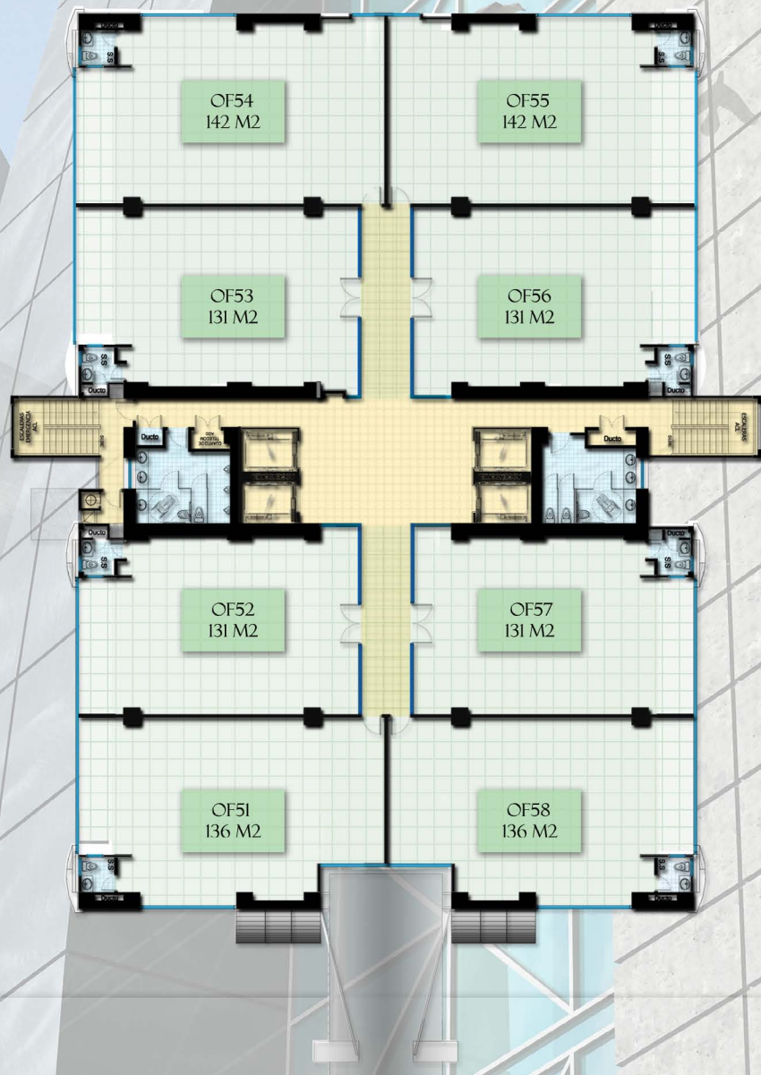
PLANTA DE DISTRIBUCION ARQUITECTONICA OFICINAS PISO 5
