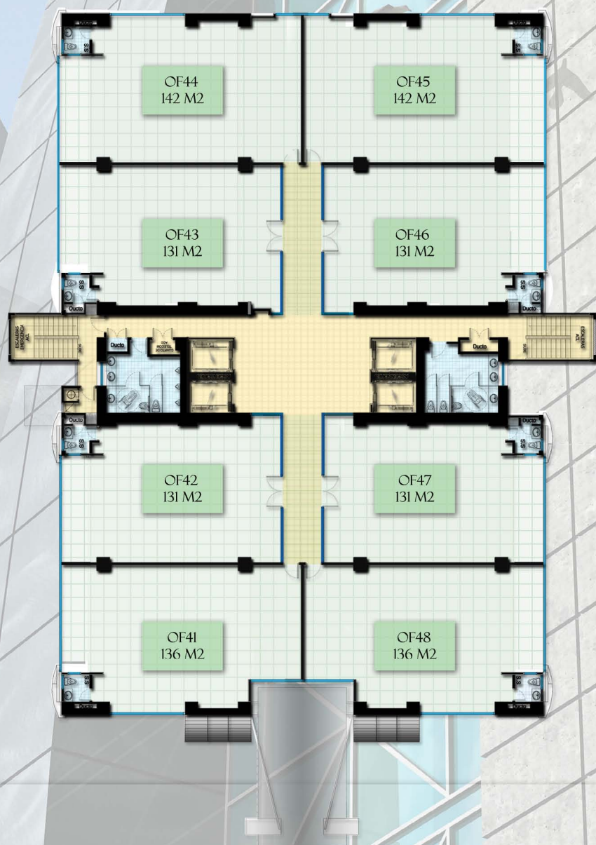
PLANTA DE DISTRIBUCION ARQUITECTONICA OFICINAS PISO 4
